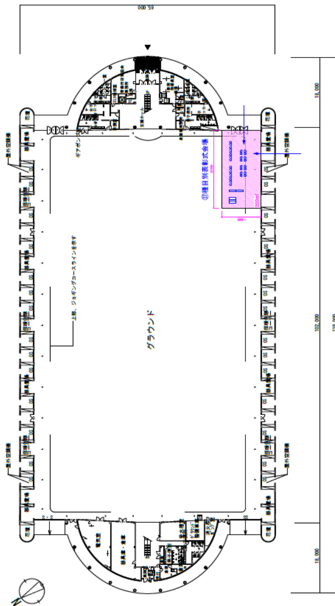
1階 平面図 S=1:600
